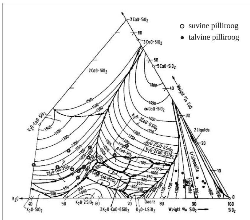
Joonis 3. Suvel ja talvel kogutud roo tuhakomponentide K_2O - CaO - SiO_2 kolmikdiagramm kantuna [5] avaldatud diagrammile. Tõlge: weight – mass, cristobalite – kristobaliit ( SiO_2 mineraal), quarz – kvarts ( SiO_2 mineraal), tridymite – tridymiit ( SiO_2 mineraal), 2Liquids – kaksikvedelik.
