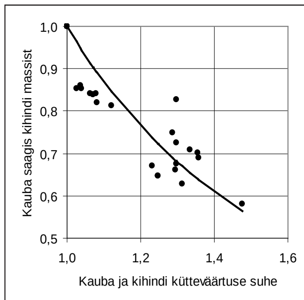
Joonis 4. Kaubapõlevkivi saagise sõltuvus põlevkivi väärastamise astmest.
