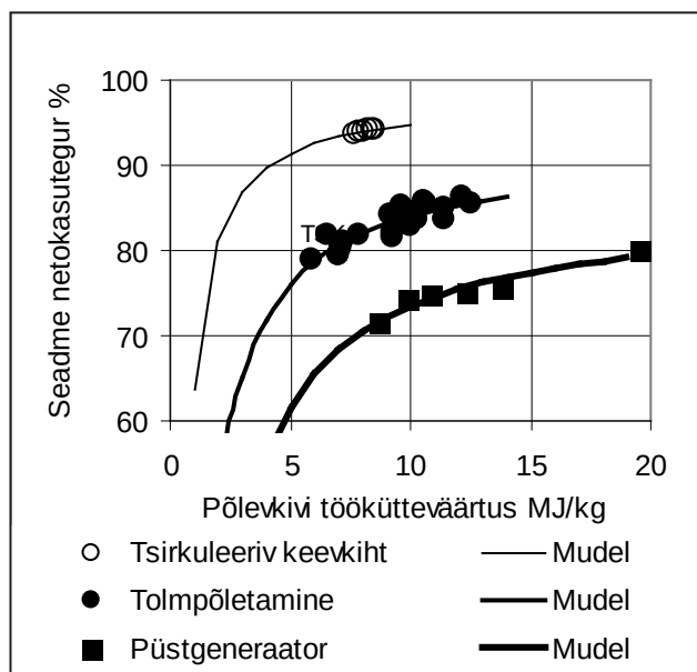
Joonis 1. Utiliseerimiseseadmete tõhususjooned – energaetilise kasuteguri sõltuvus põlevkivi kütteväärtusest.
