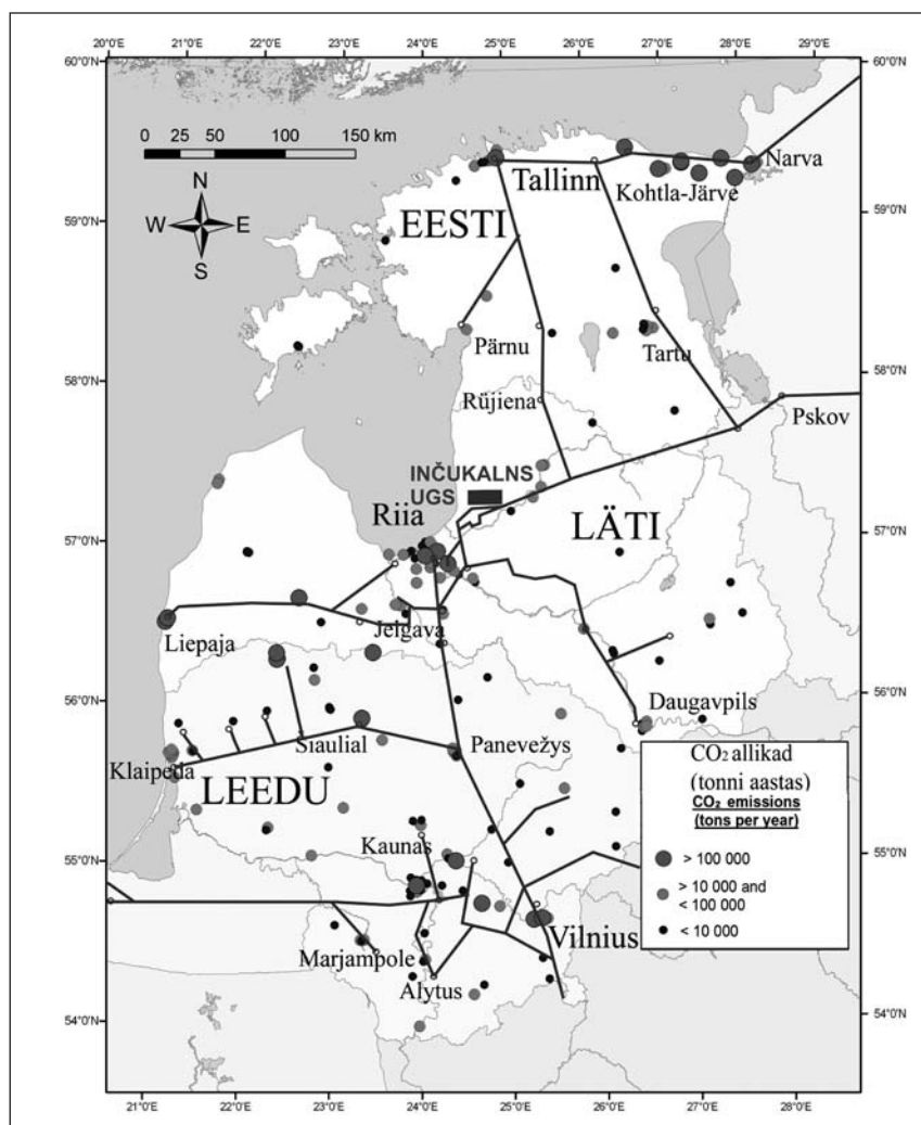
Joonis. Euroopas (European Union Emission Trading Scheme) registreeritud CO 2 allikad Eestis, Lätis ja Leedus 2005. aastal t/a. Jämedad jooned näitavad maagaasitorustikku.
