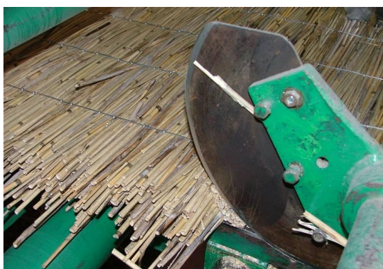
Joonis 3.50. Berger plaadi servade lõikamine (foto: M. Miljan)
