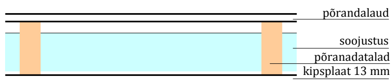
Joonis 3.33. Vahelae konstruktsioon (ET 0506-0676)
