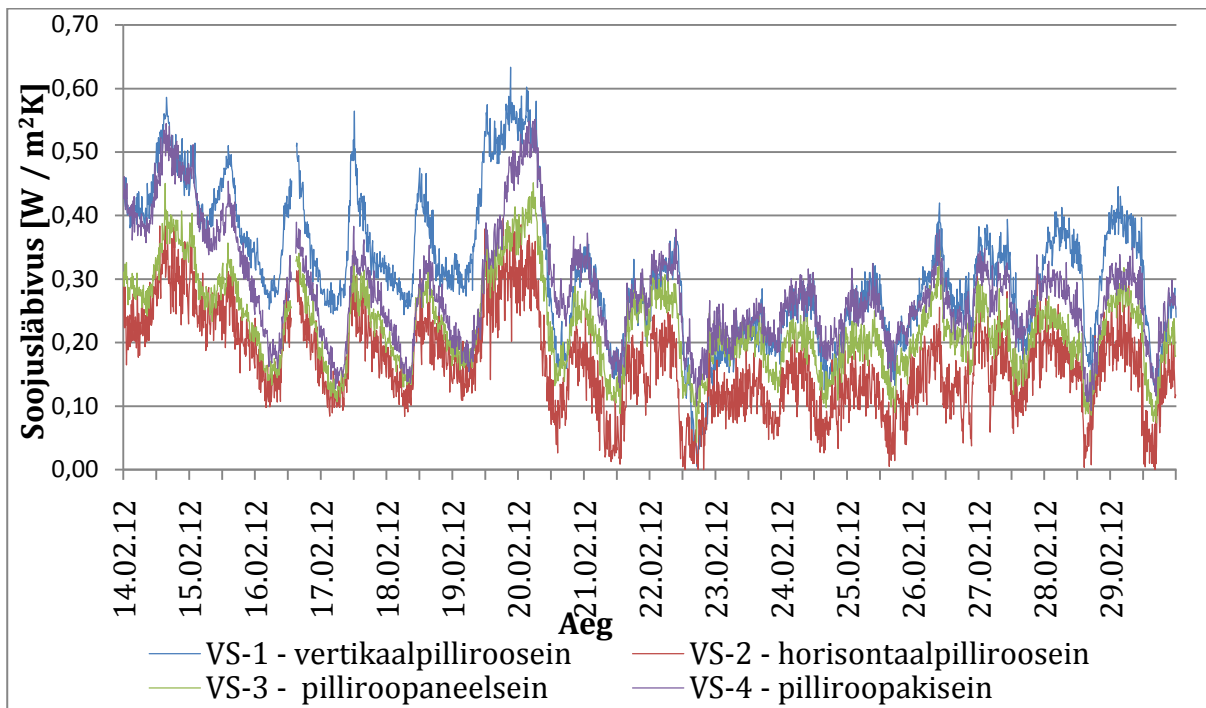
Joonis 5.3. Erinevate katseseinte soojusläbivuse muutused ajas (2012. a veebruari II pool) (Miljan, M-J. et al 2012 c)
