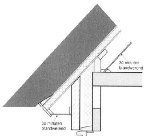
Joonis 3.41. Räästasõlme ja katusekonstruktsiooni skeem 30-minutise tulepüsivuse saavutamiseks (Brandveilige ... 2010:13)
